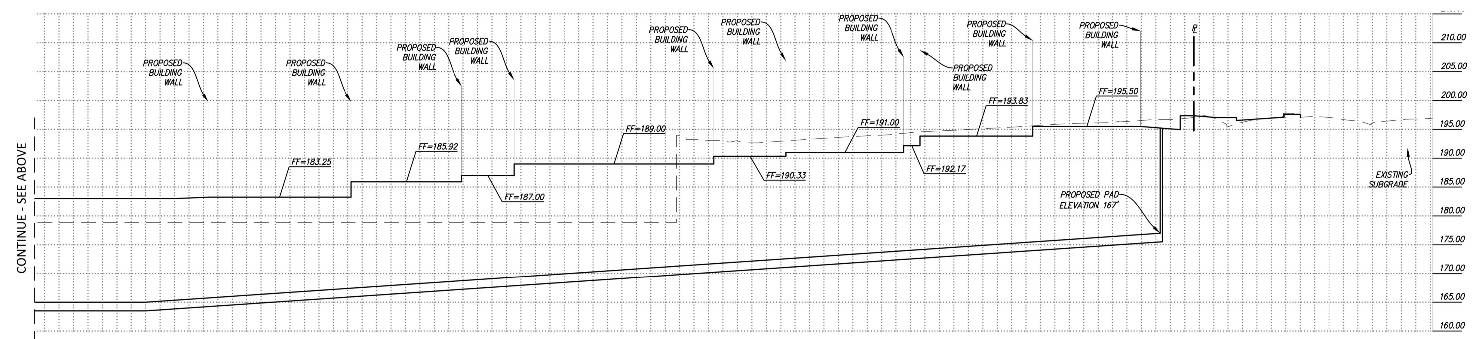
SECTION 3 HORIZ. SCALE: 1" = 40' VERT. SCALE: 1" = 10'
